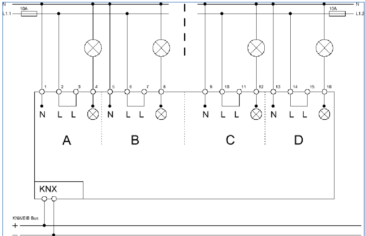
Abbildung 1: Anschluss-Schema AKD-0401.02
