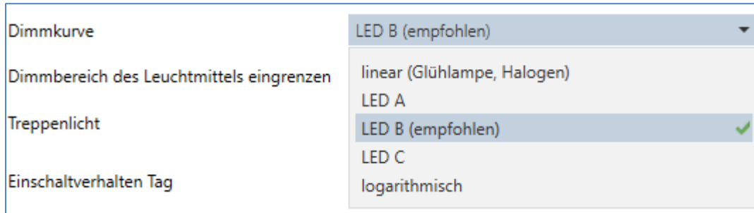
Abbildung 8: Auswahl Dimmkurve
