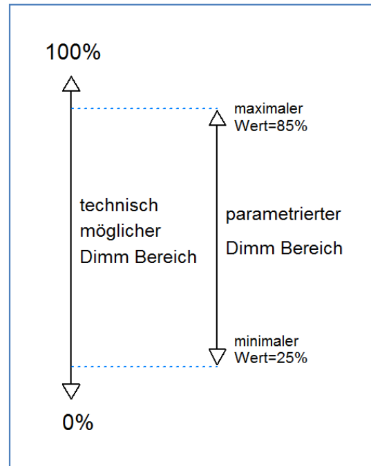
Abbildung 10: Dimmbereich eingrenzen
