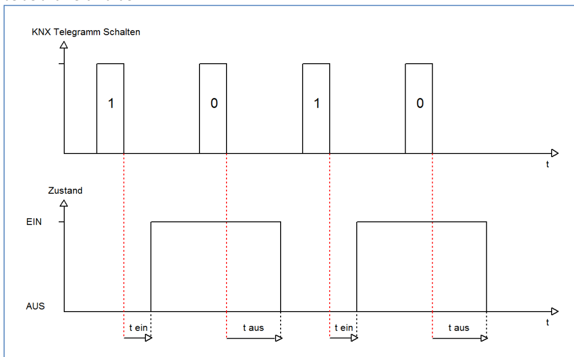
Abbildung 15: Funktionsdiagramm Ein-/Ausschaltverzögerung
