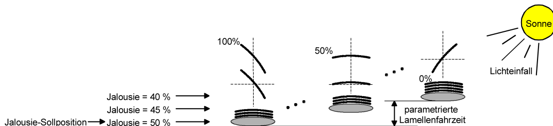
Bild 9: Beispiel für Lamellenpositionierung mit Auswirkung auf die Jalousieposition (Beispielhaft für Lamellentyp 1. Typ 2 sinngemäß gleich.)
