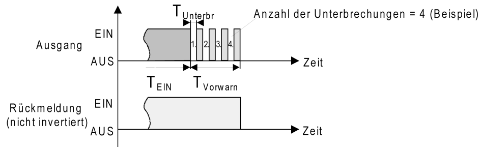
Bild 19: Die Vorwarnfunktion der Treppenhausfunktion (Beispiel)
