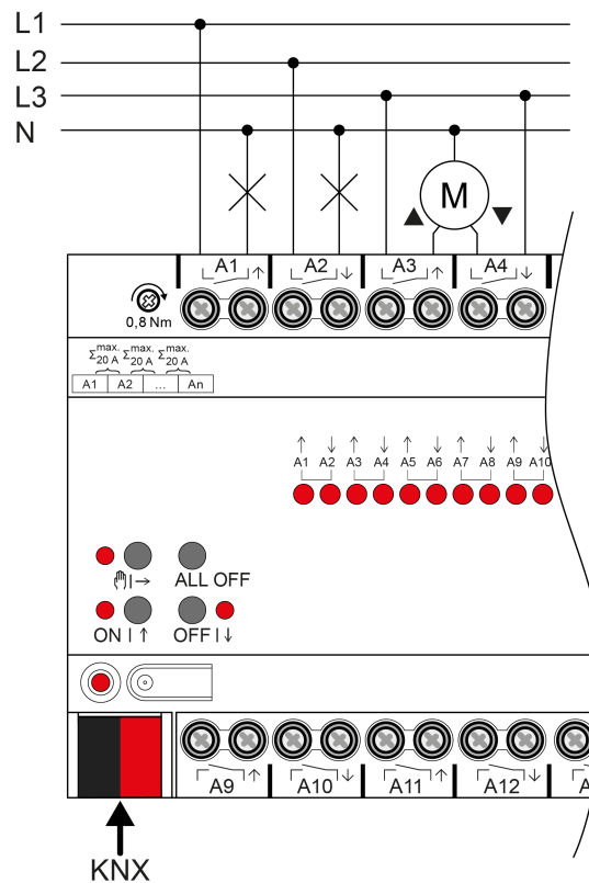
Bild 2: Geräteanschluss (Anschlussbeispiel)
