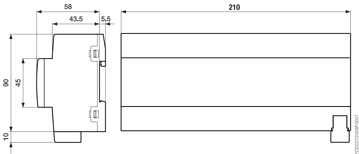
Abb. 2: Maßbild
