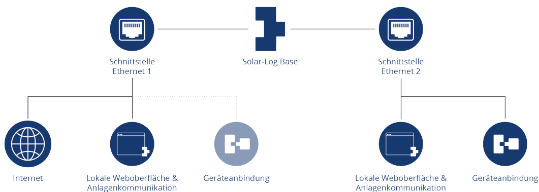
Beispiel mit Aktivierung beider Ethernet-Schnittstellen
