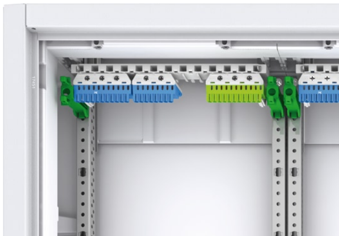
Kleinverteiler der Serie AT
