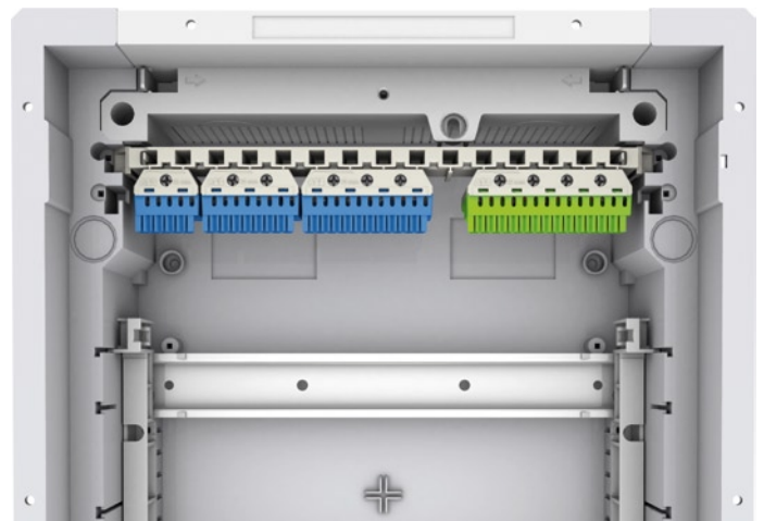
Stromkreisverteiler der Serie UK500
