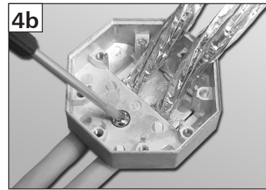
Anschlussdose 2 Port wall outlet 2 Port
