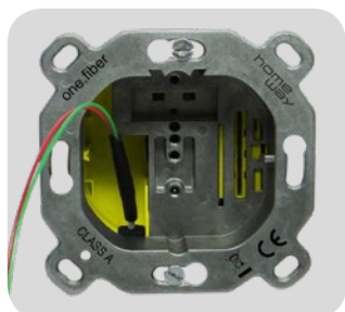
Abb.: Dose in der Wand
