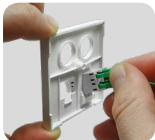
Abb.: Kupplung in die Zentralplatte stecken
