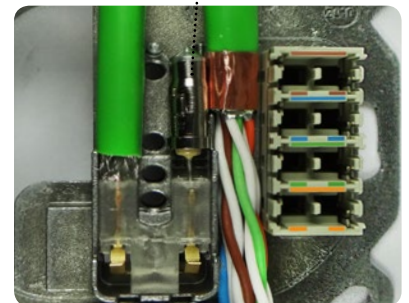
RC-Abschlusswiderstand
