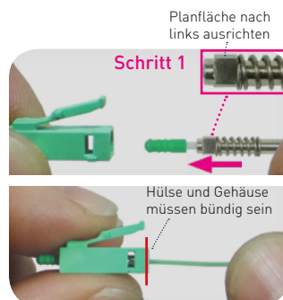
Abb.: LC/APC Steckergehäuse anbringen
