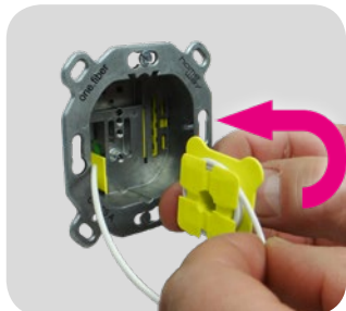
Abb.: Glasfaserkabel auf Spule wickeln
