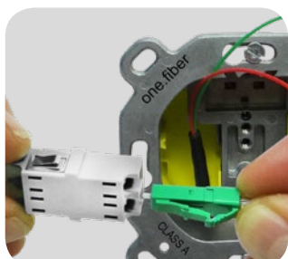
Abb.: LC/APC-Stecker in Kupplung stecken
