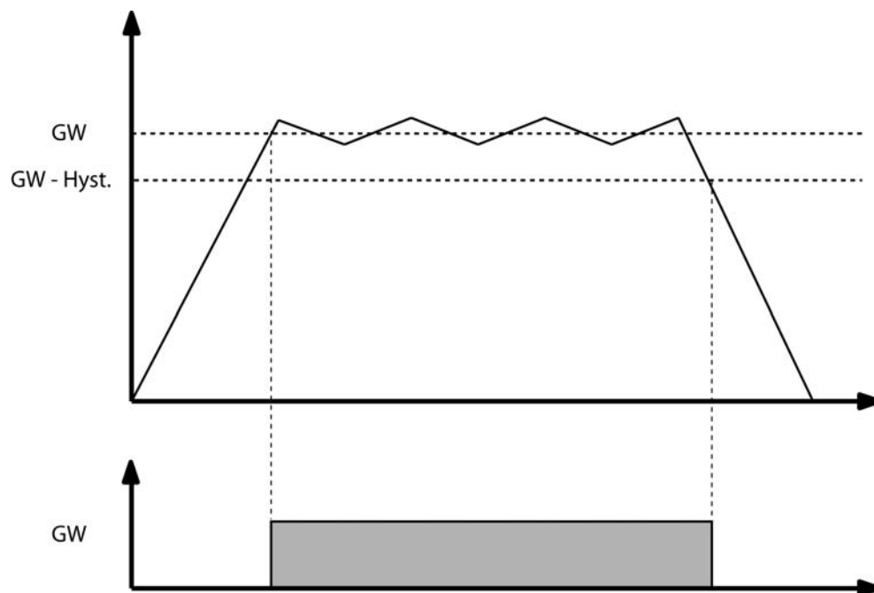
Bild 13: Schalthäufigkeit mit parametrierter Hysterese
