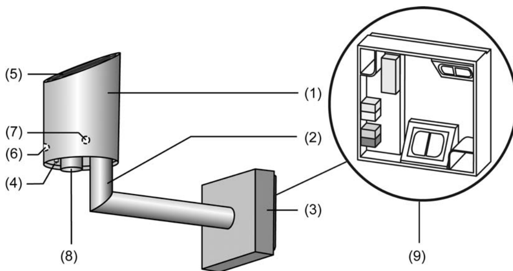
Bild 2: Wetterstation mit Klemmenkasten
