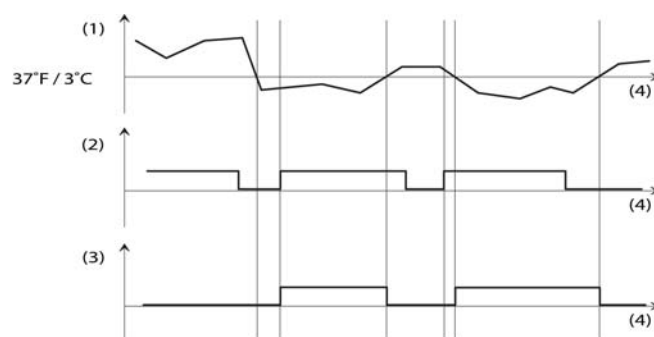
Bild 8: Vereisungsschutz in Abhängigkeit von Temperatur und Niederschlag
