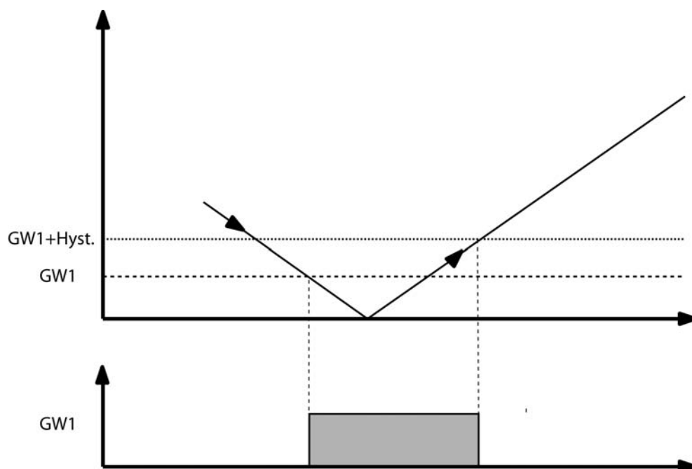
Bild 14: Aktivierung Grenzwert
