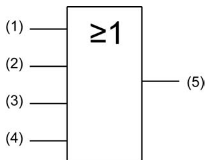
Bild 9: Verknüpfung der Signale
