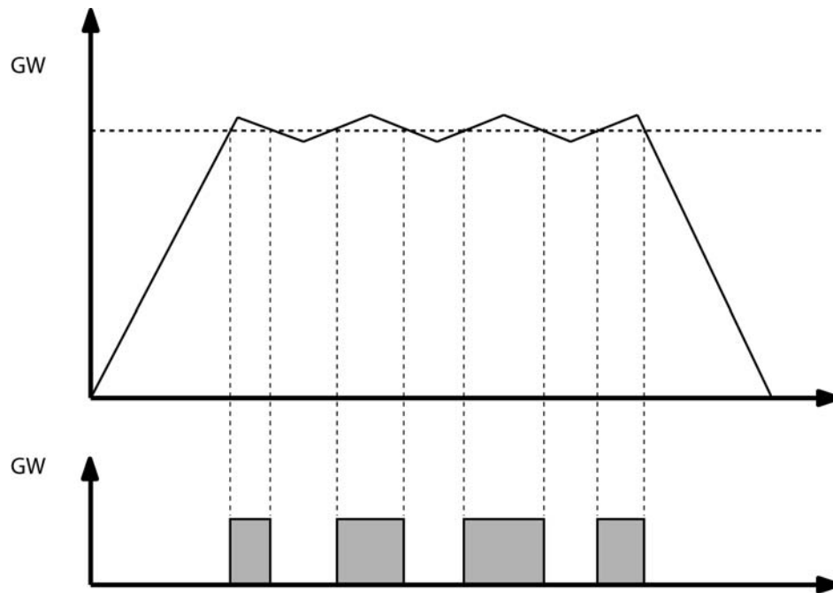
Bild 12: Schalthäufigkeit ohne Hysterese
