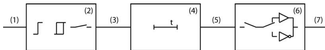
Bild 15: Blockdiagramm Ein- und Ausschaltverzögerung
