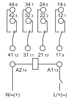
Ansteuerung über Startkontakt in der Zuleitung zu A1
