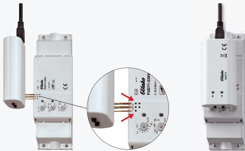
Aufstecken des Datenübertragers DAT71 auf einen Aktor der Baureihe 71.
