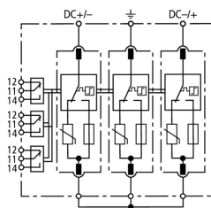
Prinzipialschaltbild DG ME YPV SCI1500 FM
