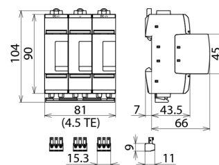
Maßbild DG ME YPV SCI1500 FM
