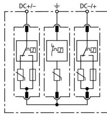
Prinzipschaltbild DG M YPV SCI 1200
