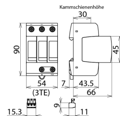
Maßbild DG M TNC 385 FM
