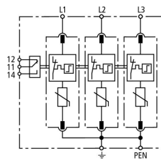
Prinzipschaltbild DG M TNC 385 FM
