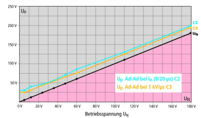
Schutzpegeldiagramm DBX U4 KT DB S 0-180
