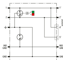
Prinzipialschaltbild DBX TC B 180
