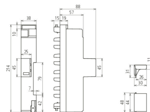
Maßbild DSH ZP 2 TNS 255
