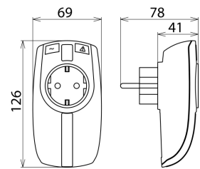
Maßbild DPRO 230
