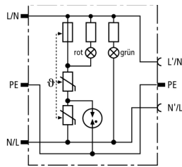
Prinzipschaltbild DPRO 230
