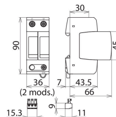
Maßbild DG MU CGD 480 3W+G
