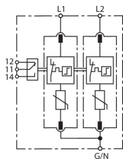
Prinzip Schaltbild DG MU CGD 480 3W+G
