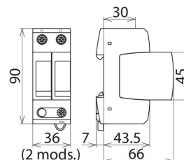
Maßbild DG MU CGD 480 3W+G
