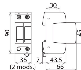
Maßbild DG MU CGD 240 3W+G
