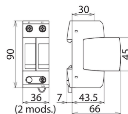
Maßbild DG MU SP 240 3W+G
