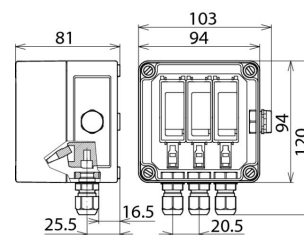
Maßbild DCU YPV SCI 1000 1M
