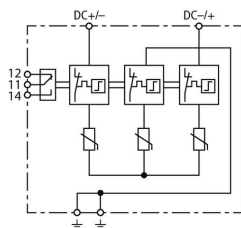
Principalschaltbild DCB YPV 1200 FM
