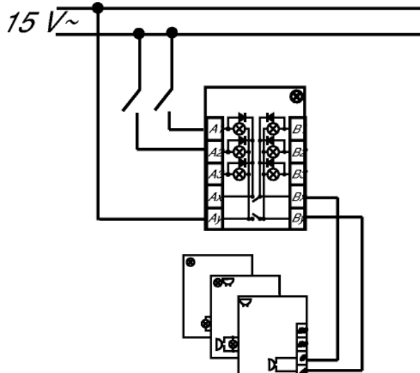
Kontrollanzeige-Einsatz 1566 U mit Gruppensignalmeldung
