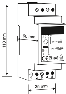
Netzteil 12 V DC/1A
