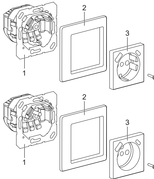
Abb. 1: Geräteaufbau
