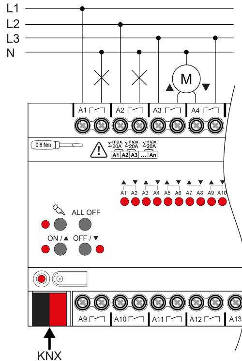
Bild 3: Geräteanschluss (Anschlussbeispiel)
