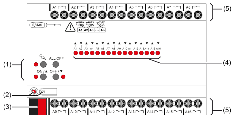
Bild 1: Geräteaufbau
