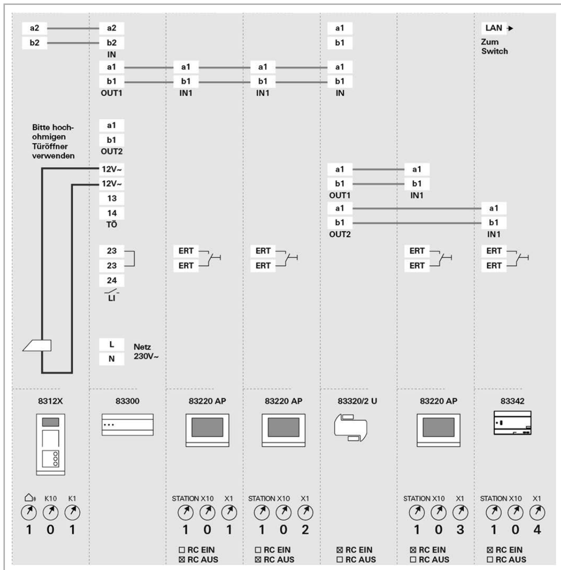
Abb. 30: Audio mit Telefon-Gateway Programmierung über ein IP-Gateway
