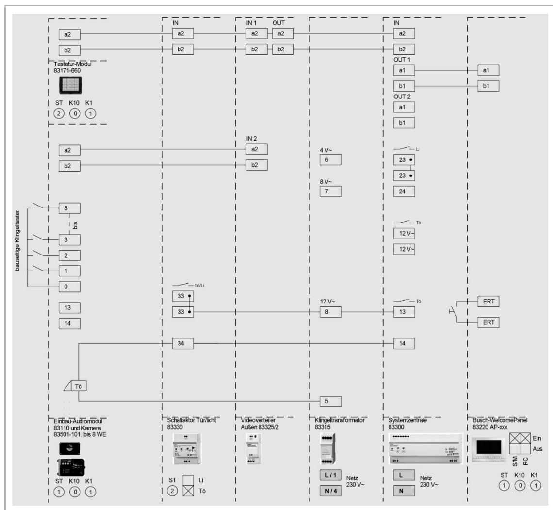
Abb. 14: Video-Außenstation mit Zutrittskontroll-Modul als Einbaukomponenten
