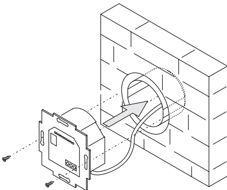
Afb. 28: Inbouwsokkel monteren
