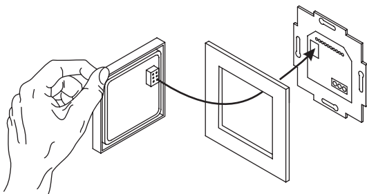
Afb. 29: Inbouwsokkel monteren
