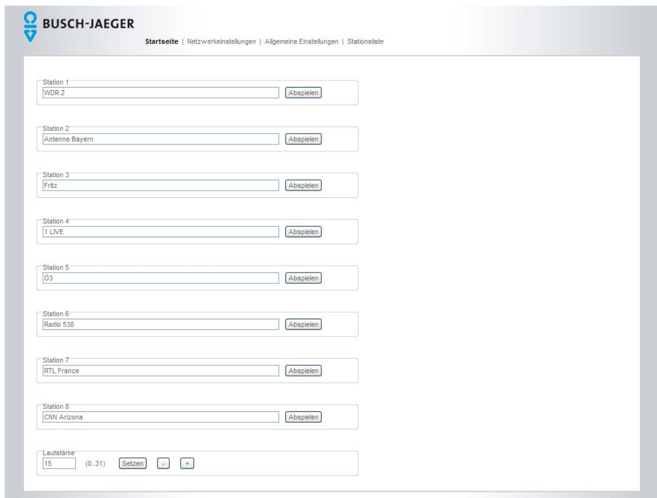
Afb. 21: Configuratiemenu “Startpagina”
