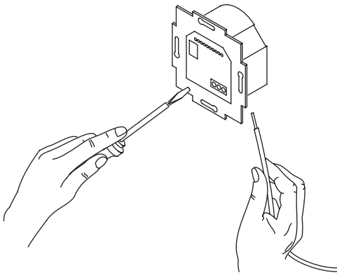
Afb. 27: Kabel aansluiten
