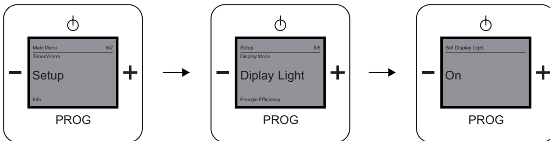
Afb. 19: Menupunt “Verlichting”
