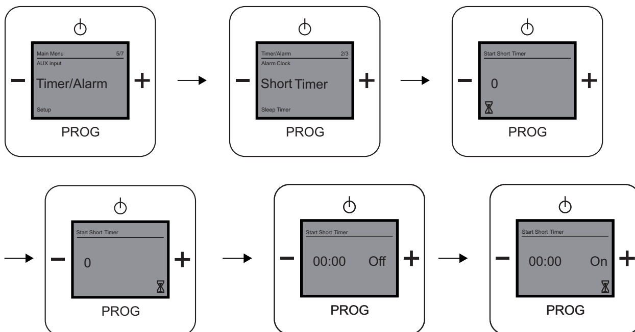
Afb. 11: Menupunt “Aftellen”
